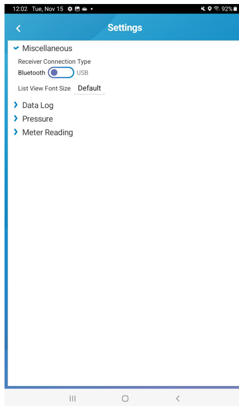
Figure 11 – Paramètres mobiles
