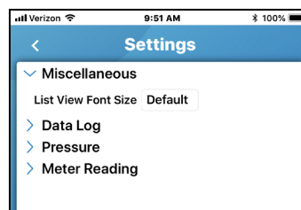
Figure 16 – Paramètres divers
