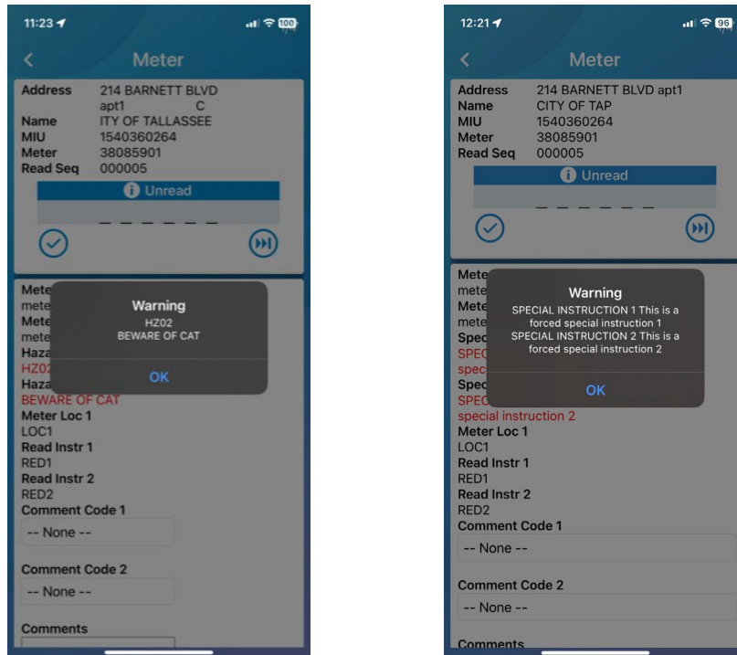
Figure 48 – Messages d'avertissement
